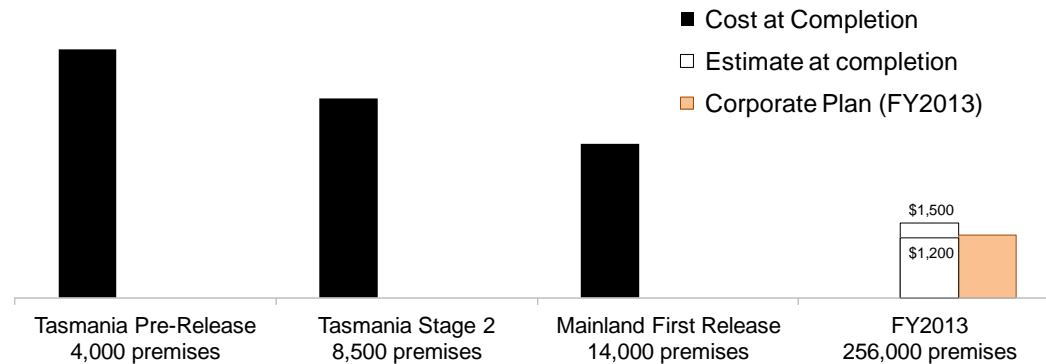
LNDN Capex Per Premise Passed
