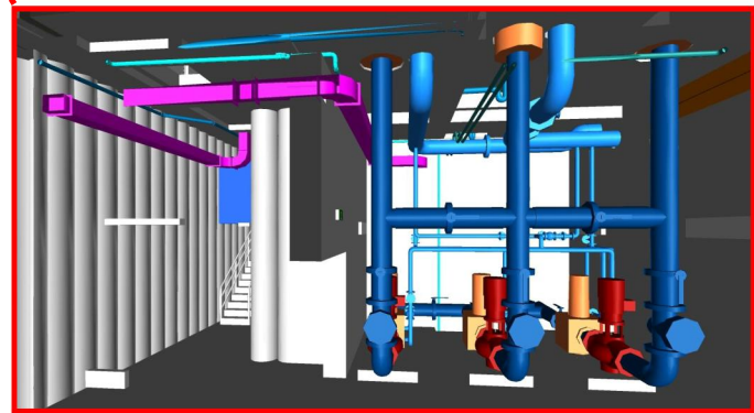
PC1 BASEMENT
