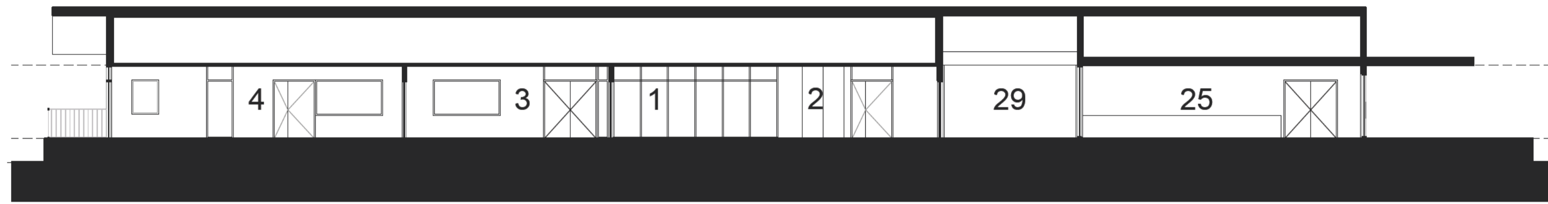
01 Section 01 -
